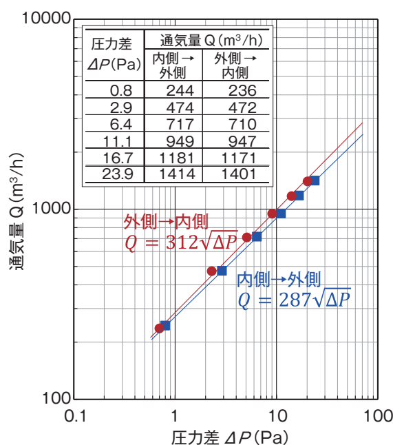
図3 通気性能試験結果
