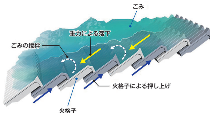
図2 F型ストーカのゴミ攪拌原理
