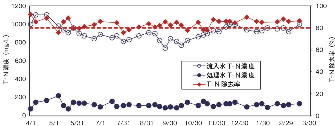
図5 T-N濃度とT-N除去率の経日変化(2019年度)
