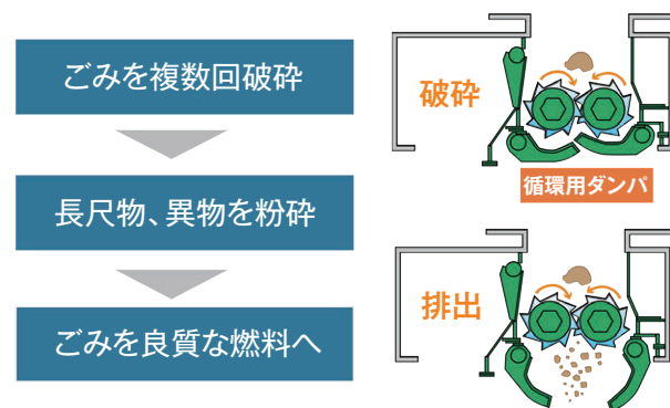
図3 循環破碎システム
