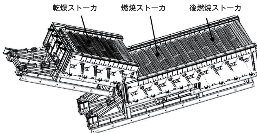
図3 開発装置(V型ストーカ)
