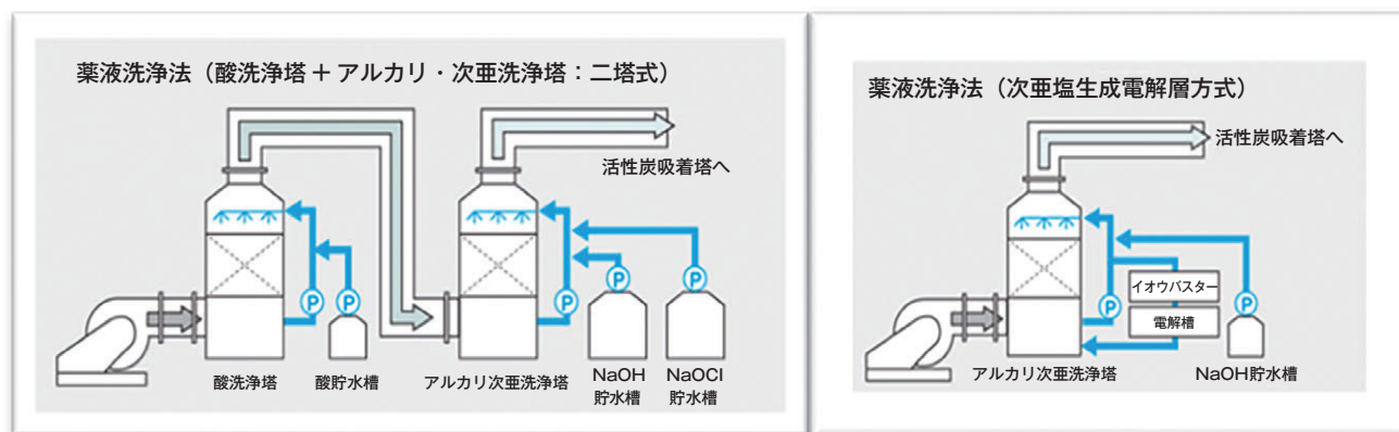
図3 従来式とISEC式の設置スペースの比較模式図
