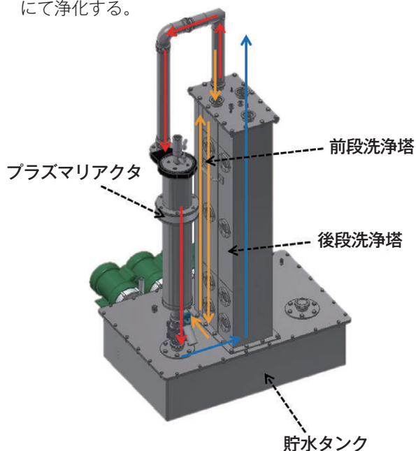
図1 装置内構成
