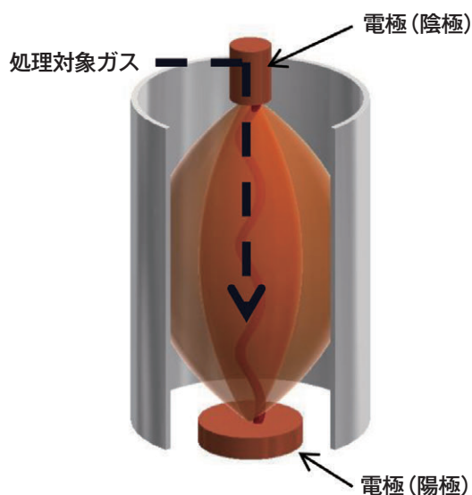
図3 ロングアーク式プラズマ
