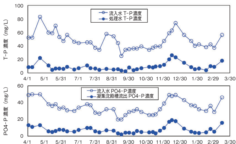
図7 りん濃度の経日変化(2019年度)
