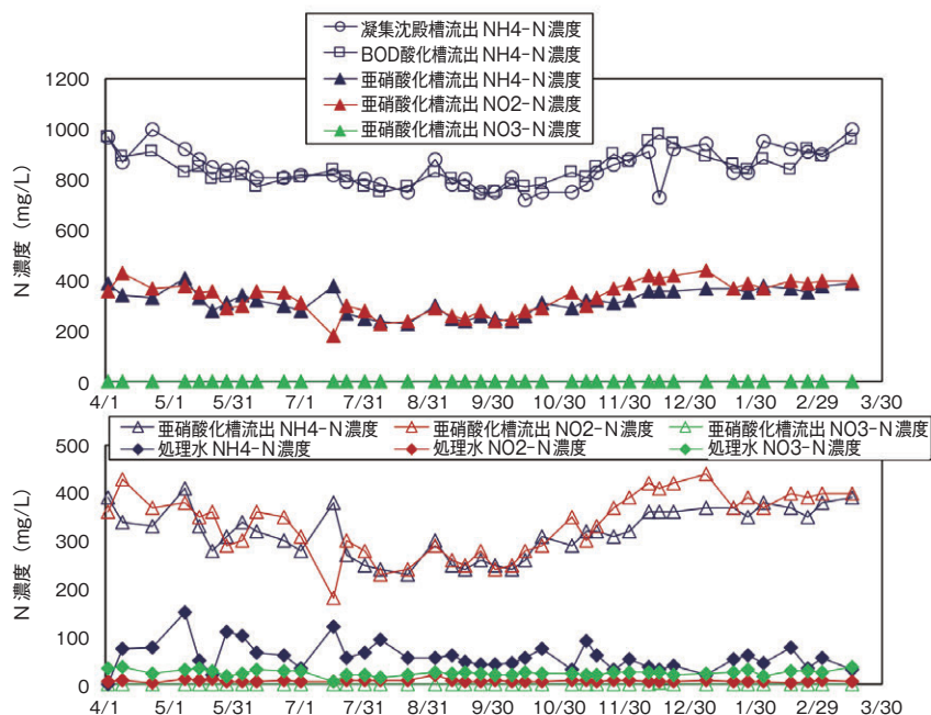
図6 各態窒素の挙動(2019年度)
